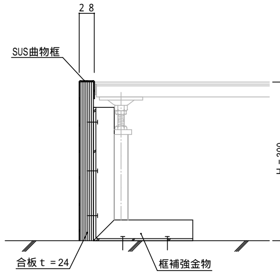
断面図 S = 1 : 5
