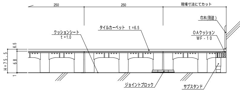
断面図 S = 1 : 5
